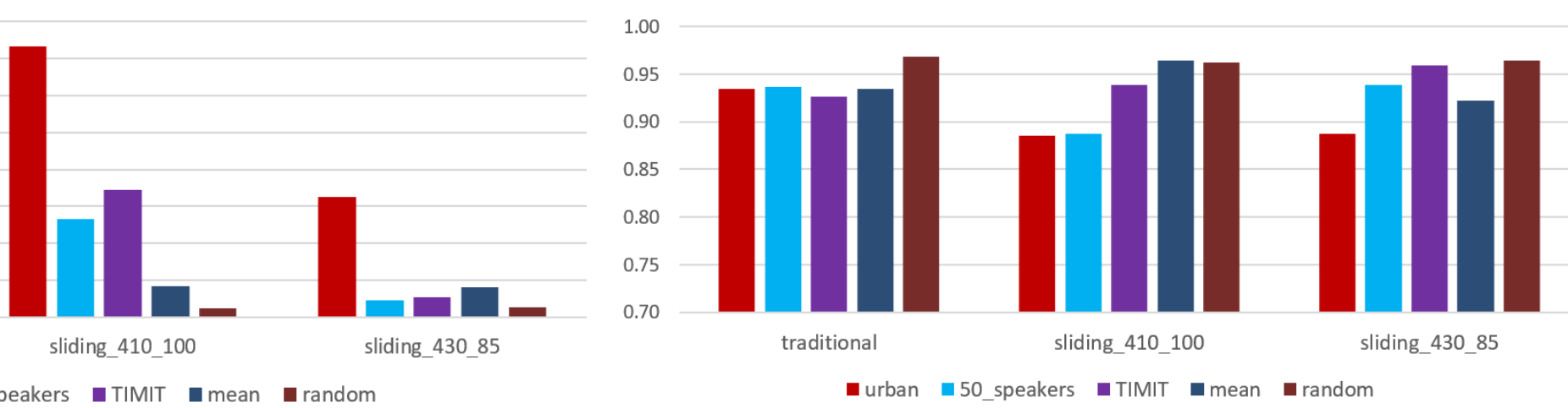
圖 5-22 50 speakers 目標模型以不同音訊作為初始化樣本的攻擊耗時(圖 5-22)與置信度(圖 5-23)
