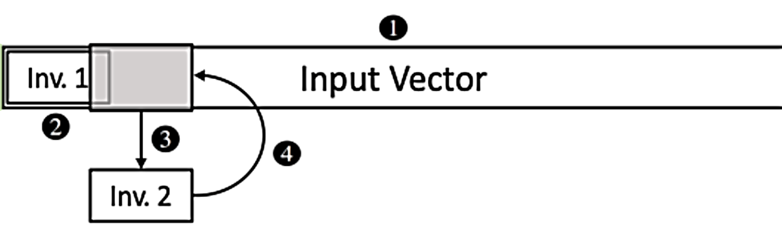
圖3-4：滑動攻擊法之攻擊示例圖
