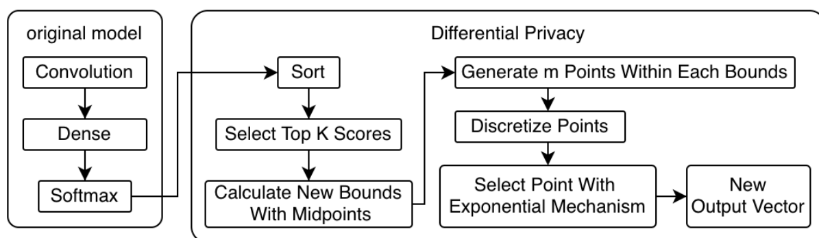
圖 3-5：差分隱私算法流程圖
