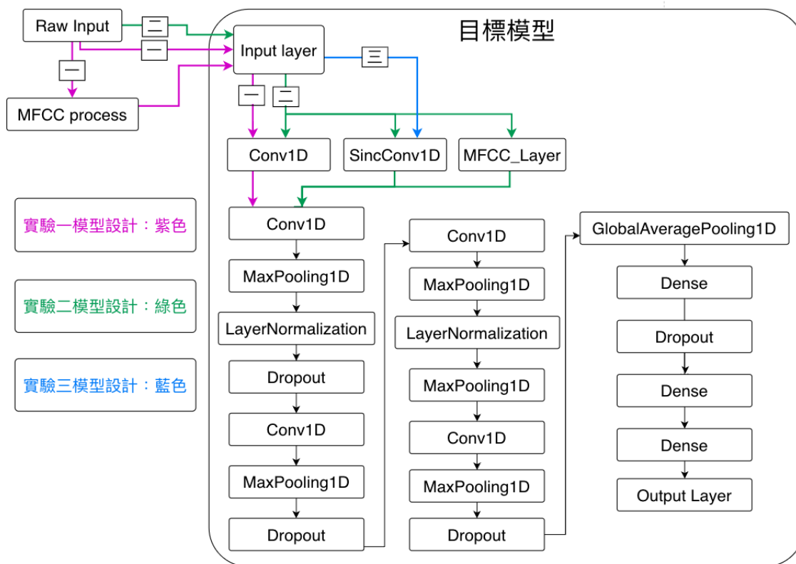
圖 3-3：實驗一、二和三語音模型訓練架構
