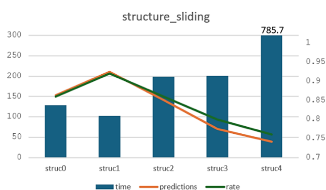
圖 4-16-2：不同模型複雜度的滑動攻擊耗時
