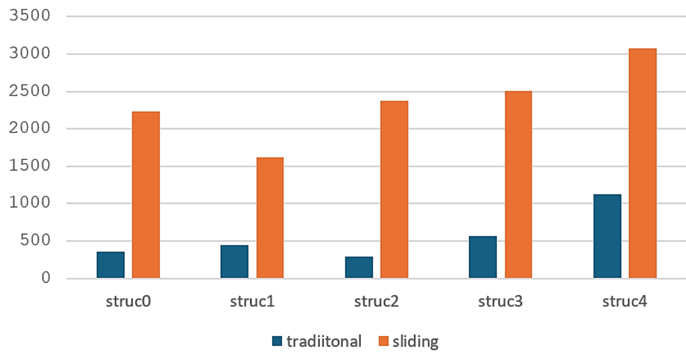
圖 5-20：滑動攻擊的不同模型複雜度攻擊結果分析
