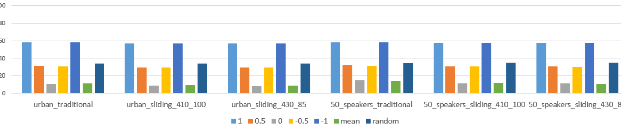
圖 5-10：SincNet 特徵擷取架構之目標模型攻擊結果與原始樣本的差異
