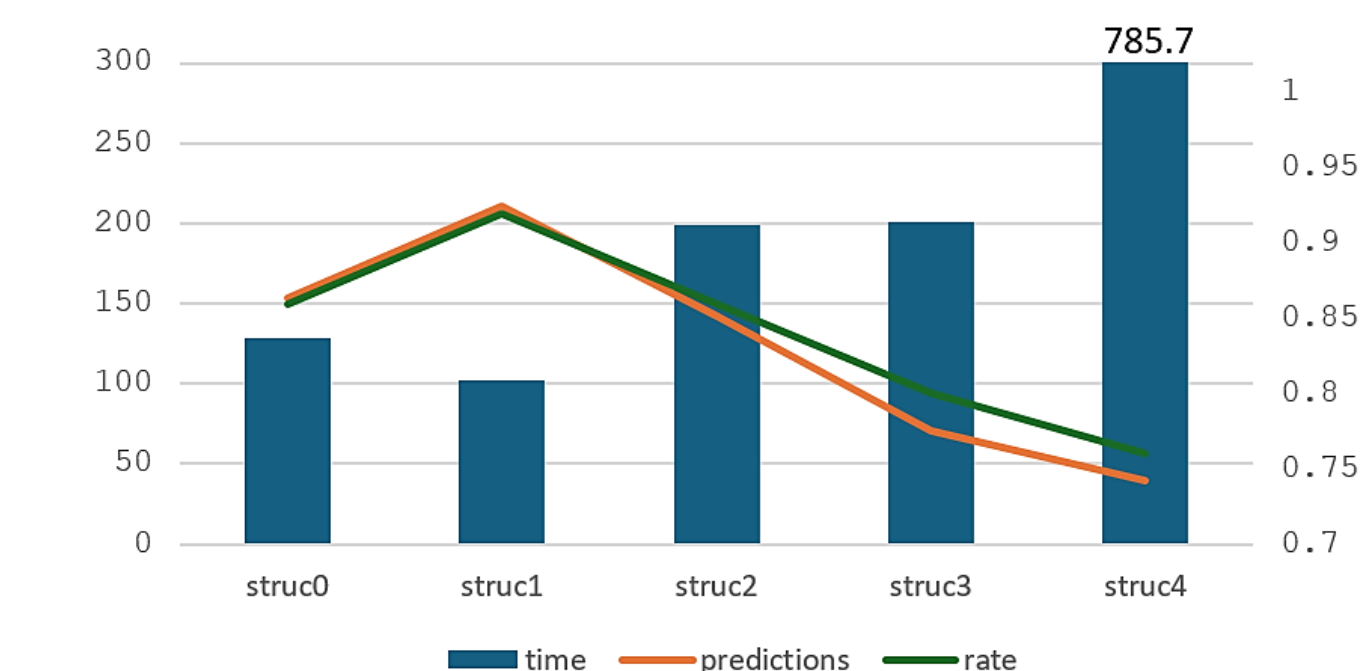
圖 5-20：滑動攻擊的不同模型複雜度攻擊結果分析
