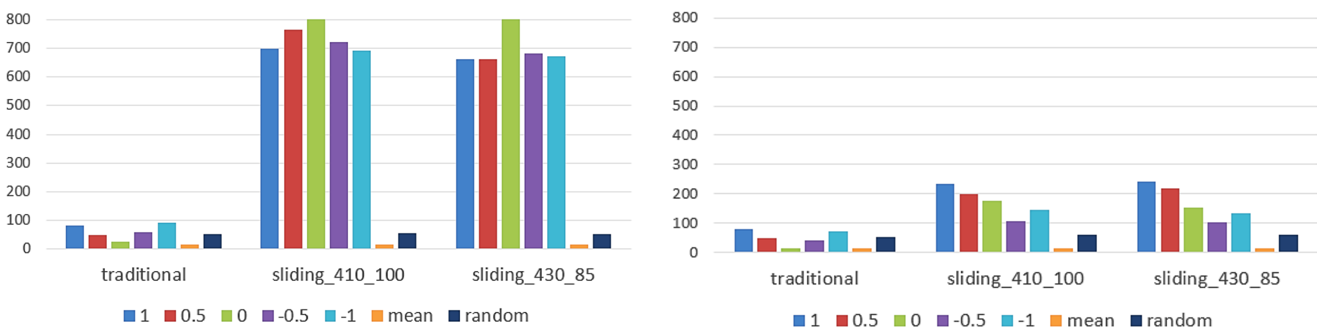
圖 5-1：以 Raw 格式輸入 50 speakers 資料 攻擊結果與原始樣本的差異
