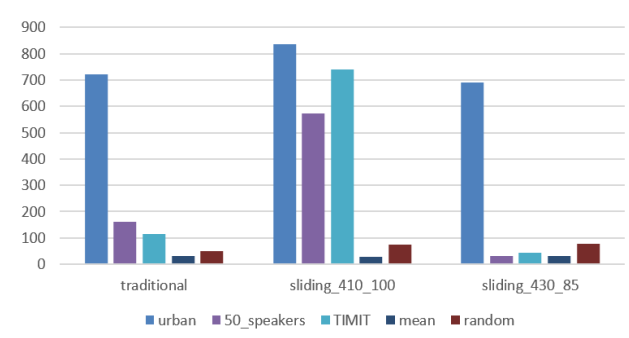
圖 4-17-5：50 speakers 目標模型以不同音訊作為初始化樣本的攻擊結果與原始樣本的距離
