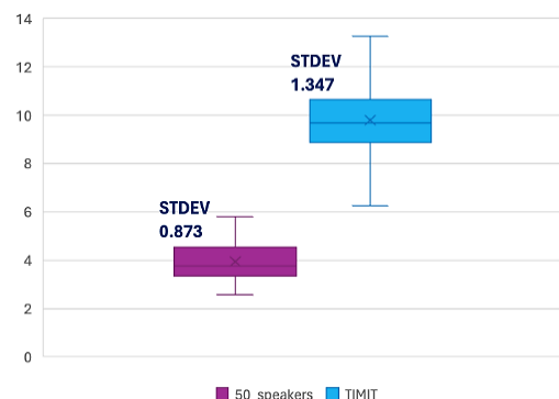
圖 4-14：資料集中不同類別樣本的差異
