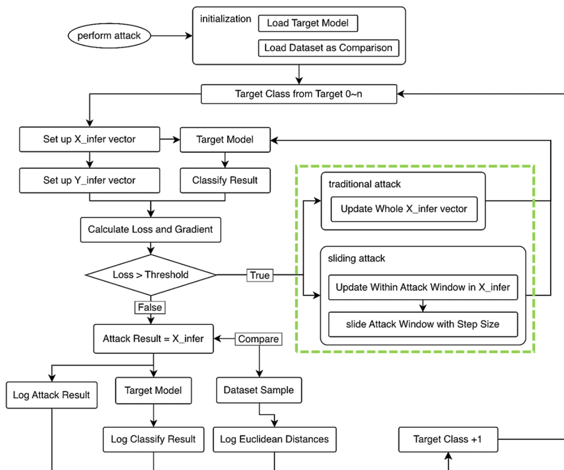
圖 3-6：逆向攻擊演算法攻擊流程圖
