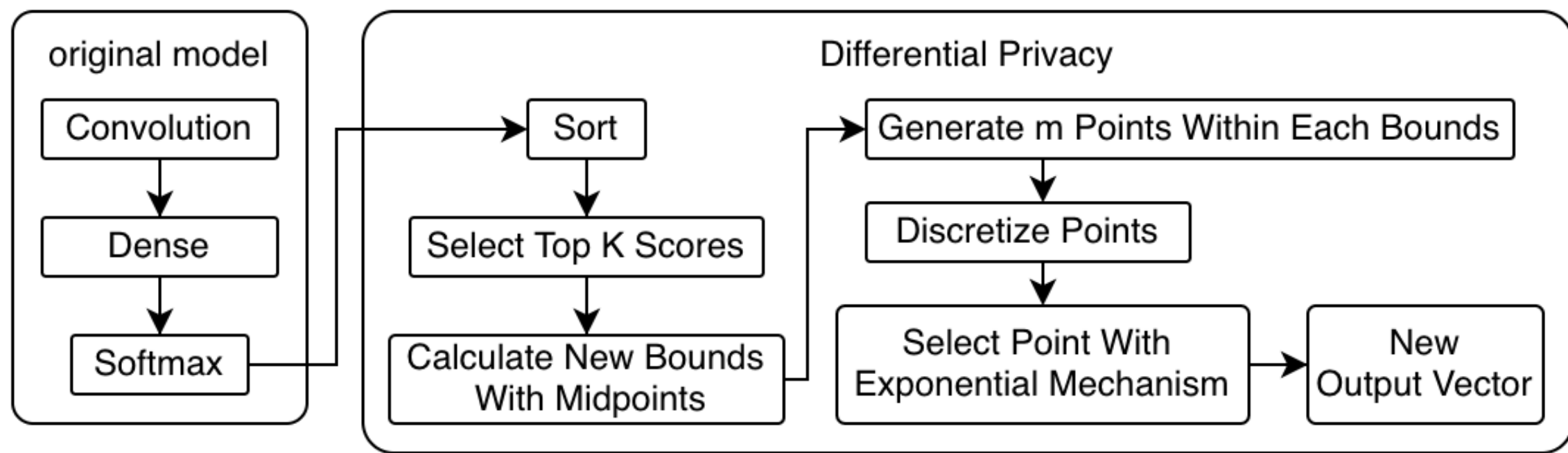
圖5-27：差分隱私防禦算法架構
