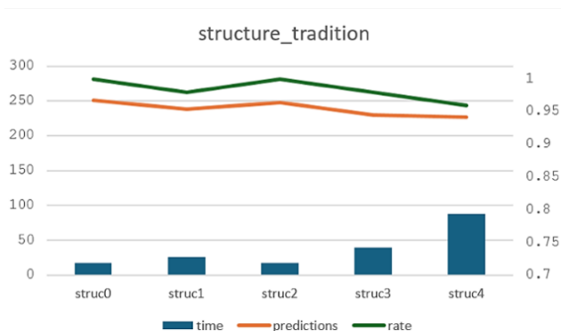
圖 4-16-1：不同模型複雜度的傳統攻擊耗時
