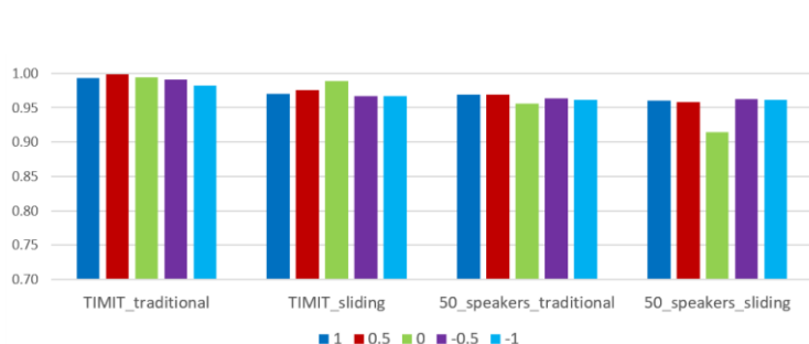
圖 4-13-1：不同人聲資料集攻擊置信度分數
