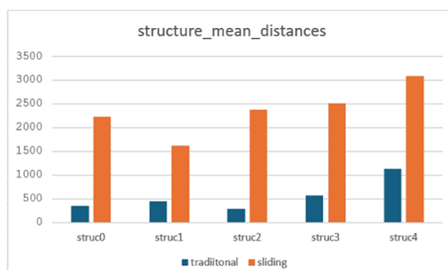
圖 4-16-3：不同模型複雜度的攻擊結果與資料集原始樣本的距離
