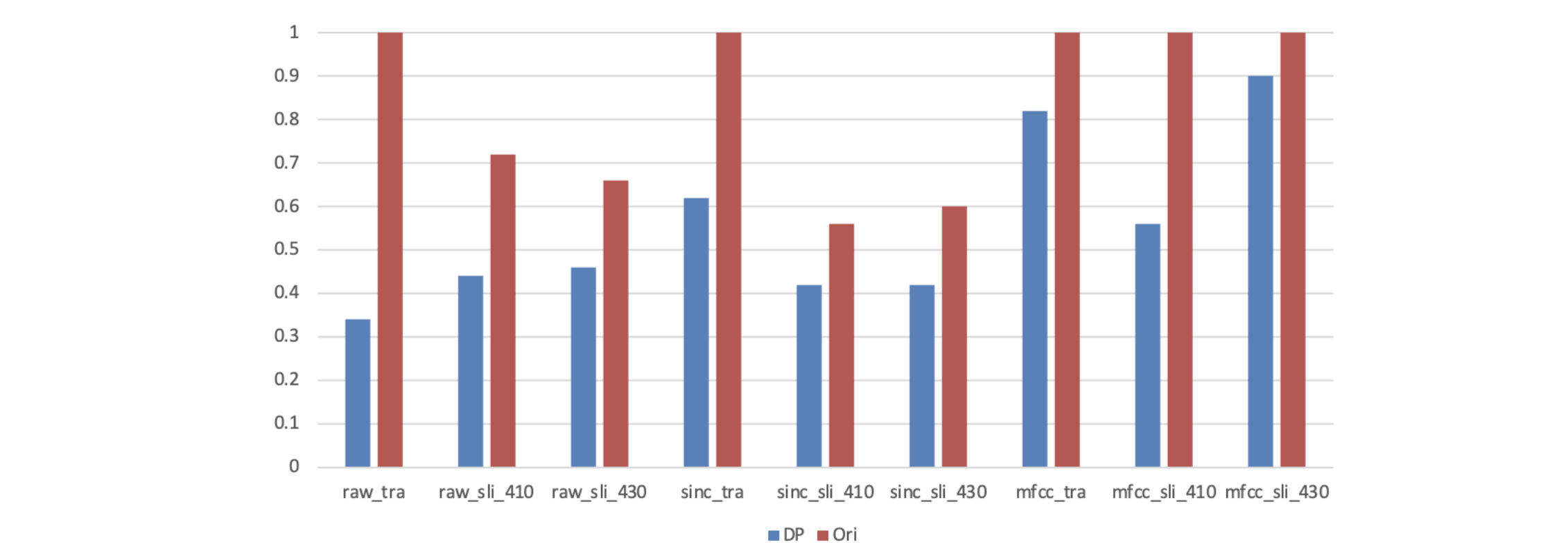
圖 5-30：差分隱私模型與原模型的攻擊成功率
