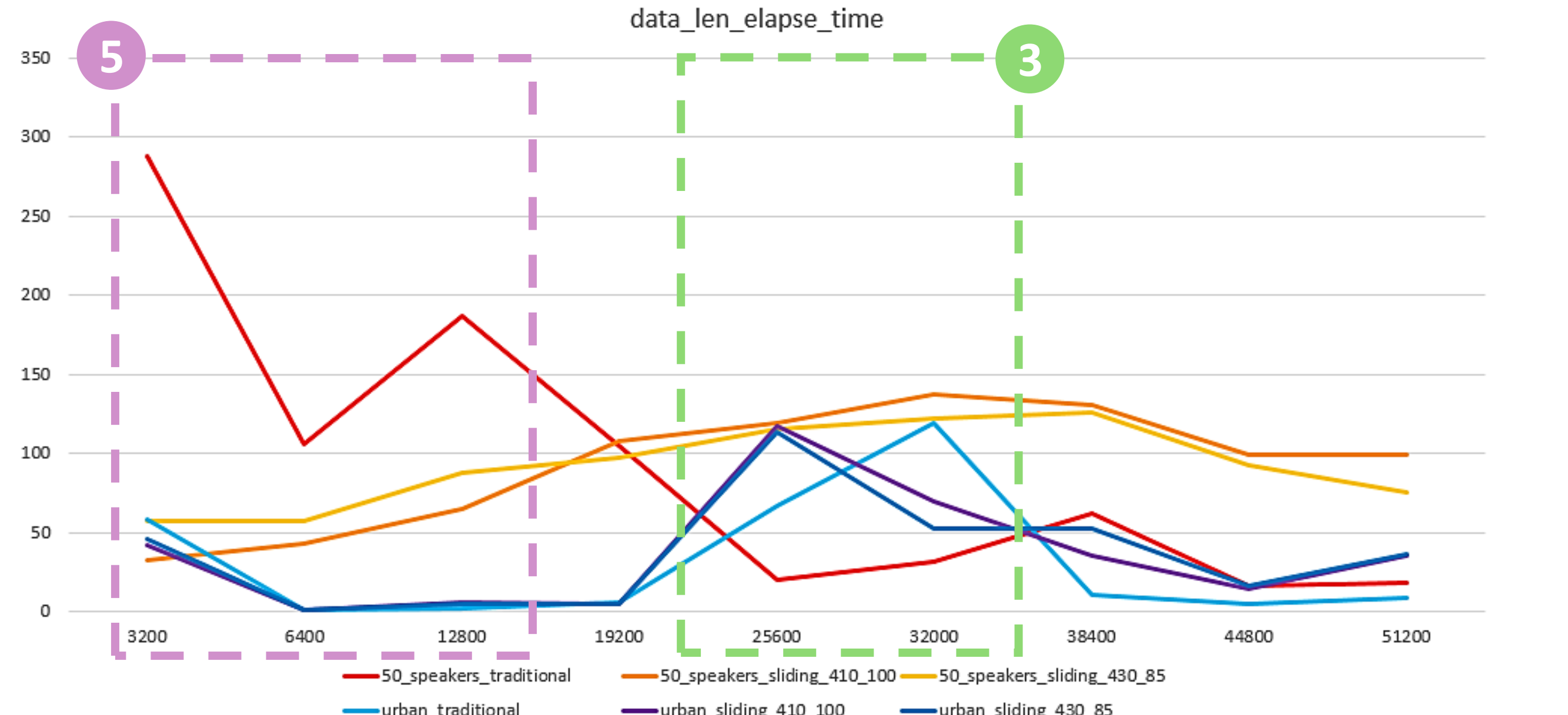
圖 5-16：不同採樣長度的模型攻擊耗時
