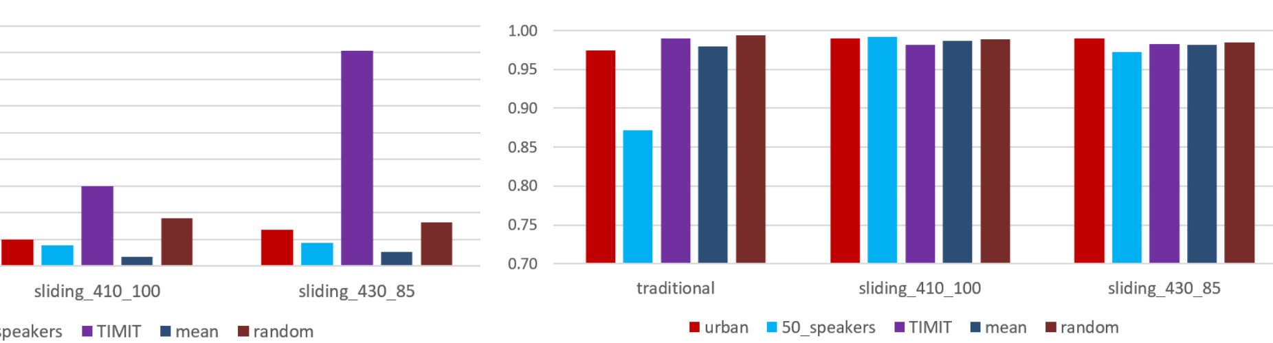
圖 5-24 urban 目標模型以不同音訊作為初始化樣本的攻擊耗時(圖 5-24)與置信度(圖 5-25)
