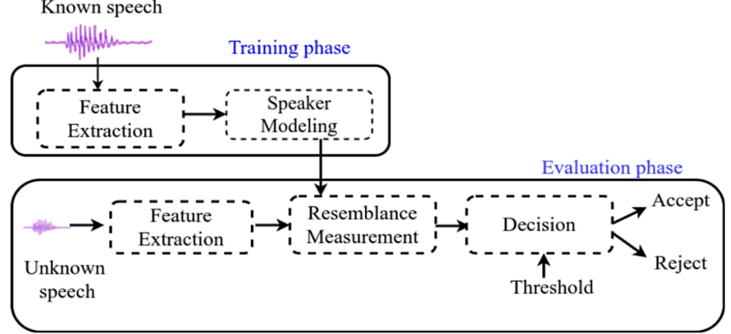
圖3-1：語者識別系統架構圖
