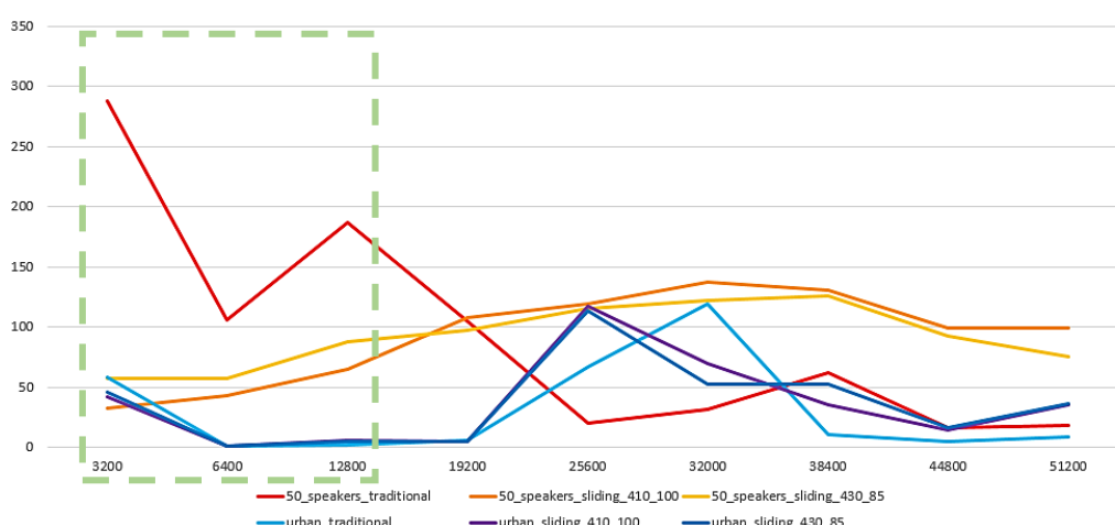
圖 4-15-1：不同採樣長度的模型攻擊耗時
