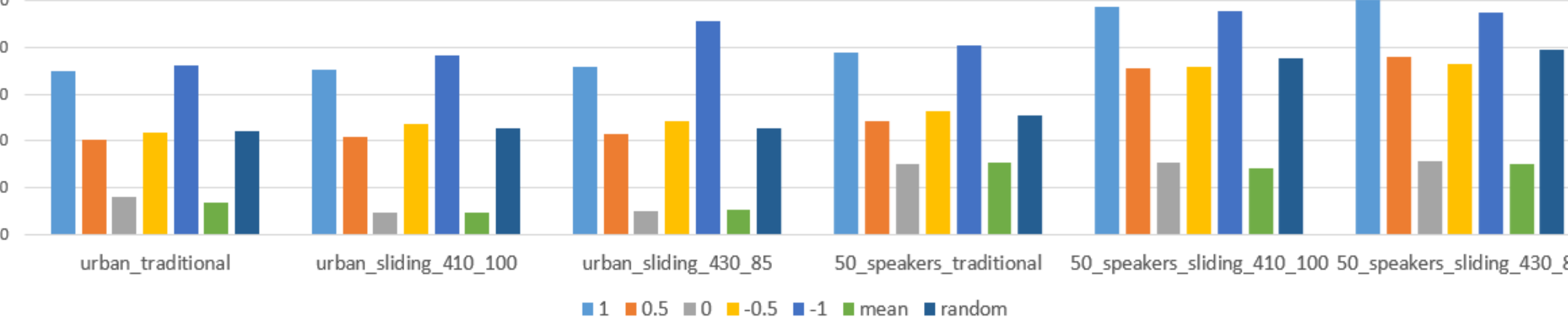
圖 5-9：MFCC 特徵擷取架構之目標模型攻擊結果與原始樣本的差異
