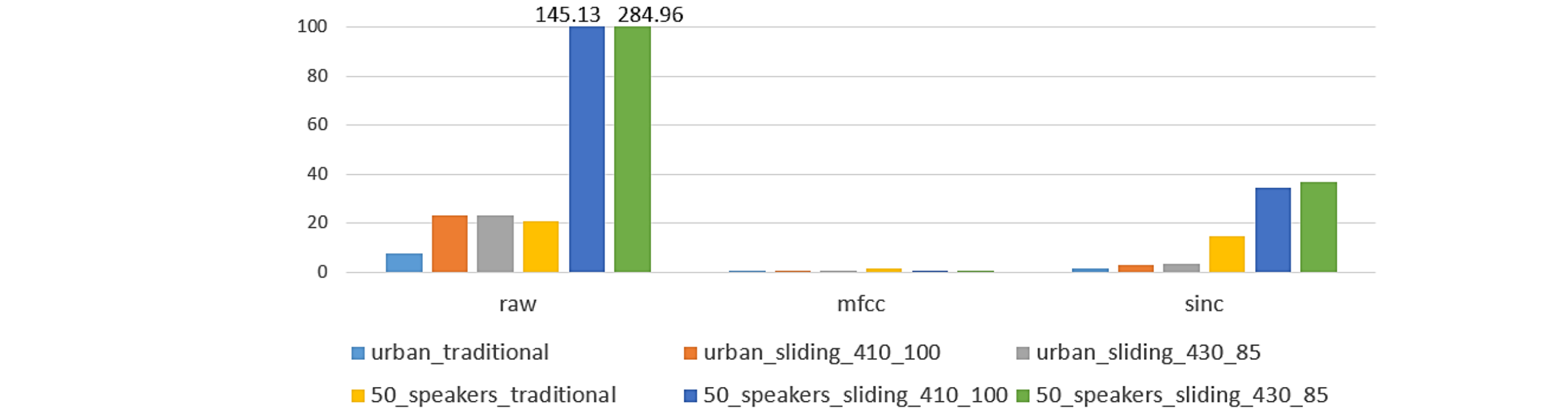
圖 5-8：不同特徵擷取架構之目標模型的攻擊耗時
