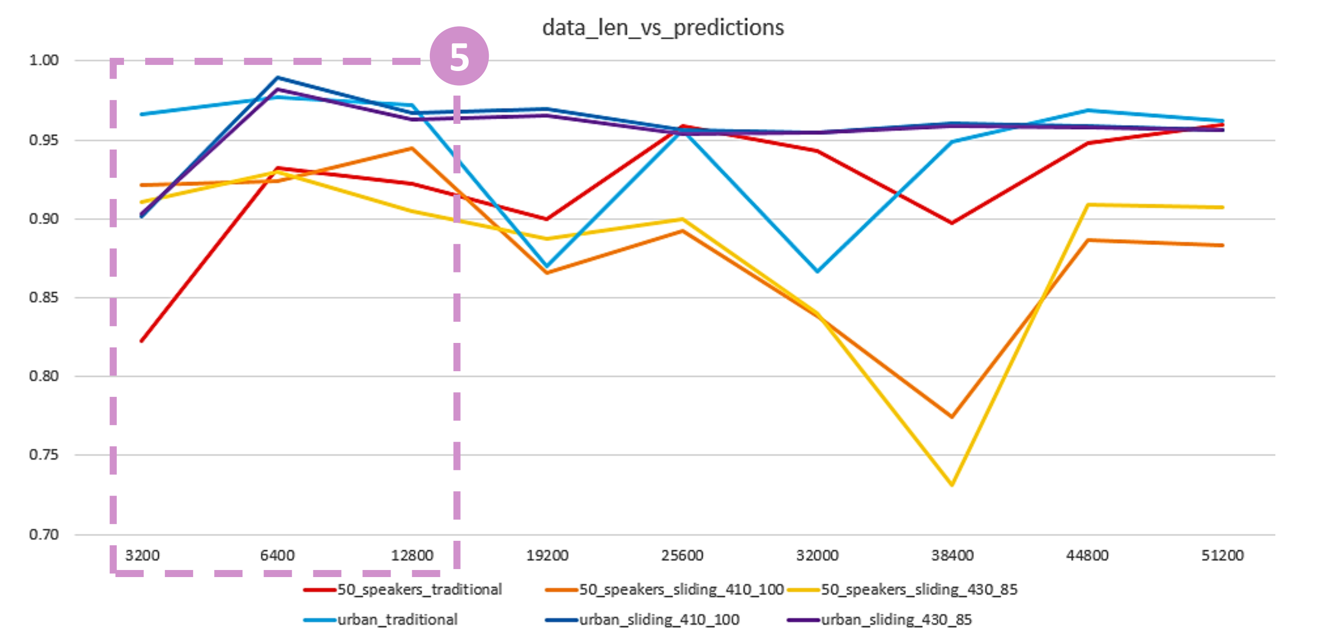
圖 5-18：不同採樣長度的模型攻擊置信度分數
