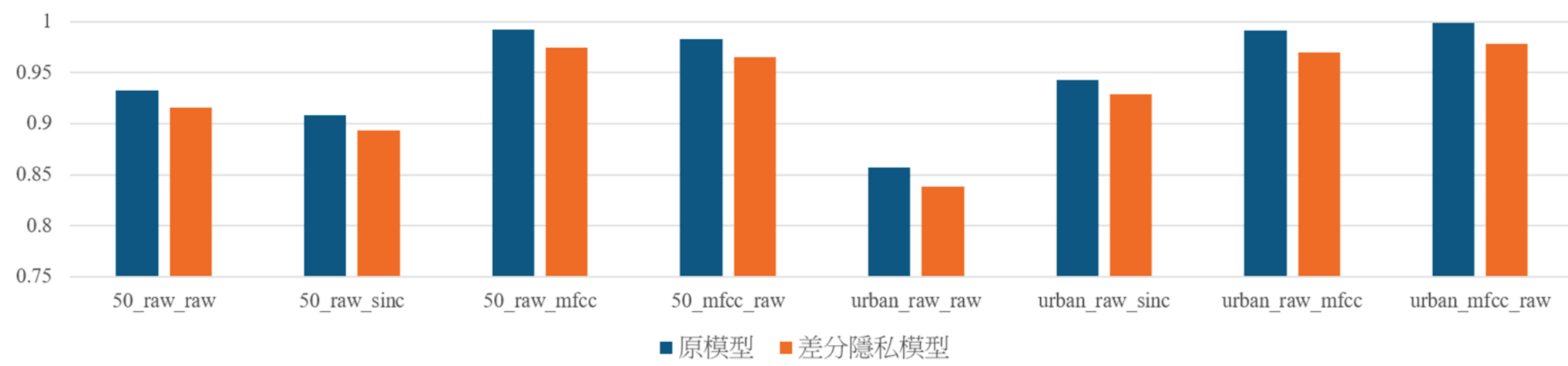
圖5-28：差分隱私模型與原模型的分類性能(accuracy)比較
