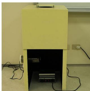
自製發煙點測定裝置 (A. O. C. S. 之規格)
