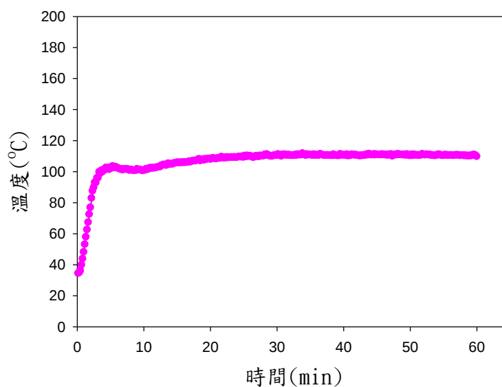
圖 16 第一代溫控裝置之溫度變化
