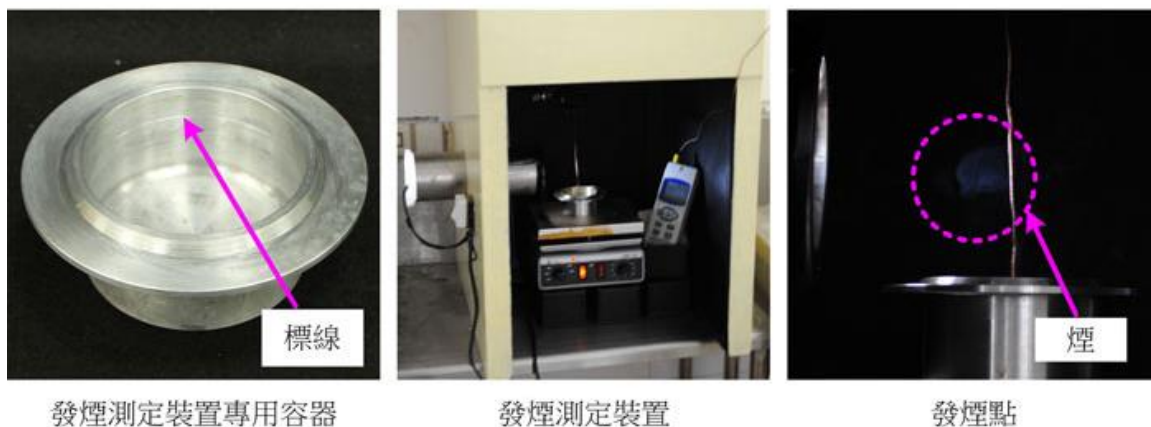
圖 29 發煙點測定裝置
