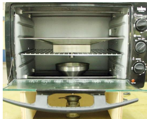
B. 組裝完成之集油裝置
