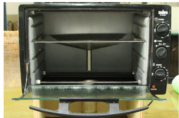
B. 組裝完成之集油裝置
