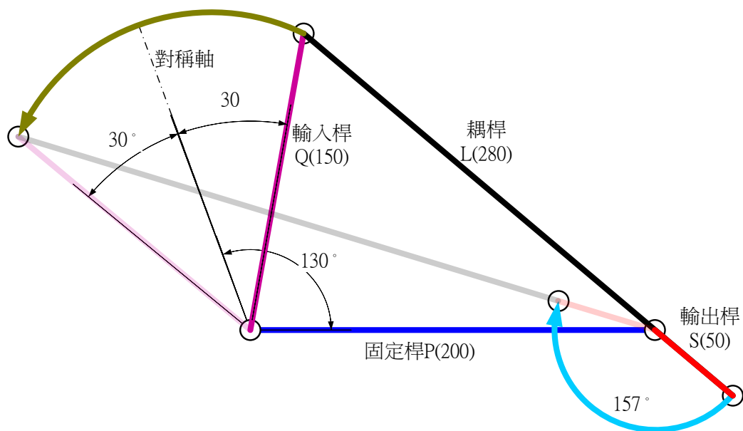
圖 9 輸入桿逆時針方向操作之輸出模擬
