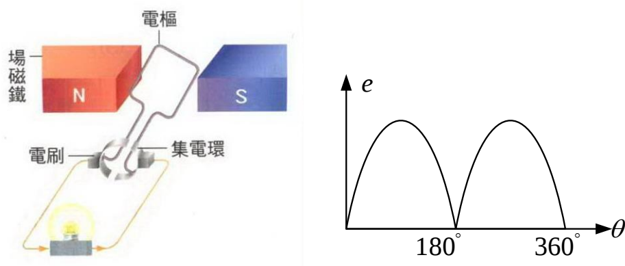
圖 5 單匝基本直流發電機 (左)基本構造 (右) 輸出波形
