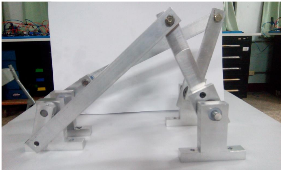
圖 23 搖桿曲柄四連桿驅動機構組裝
