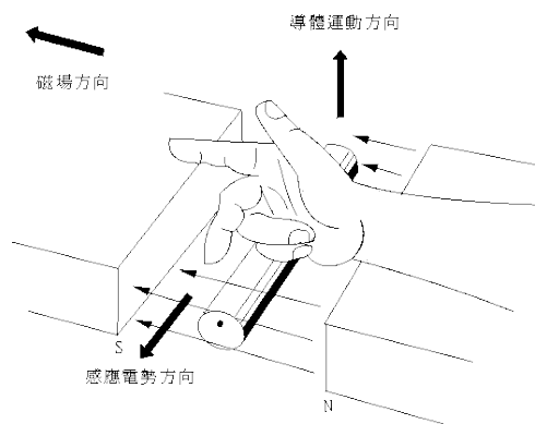
圖 4 佛萊銘右手定則
