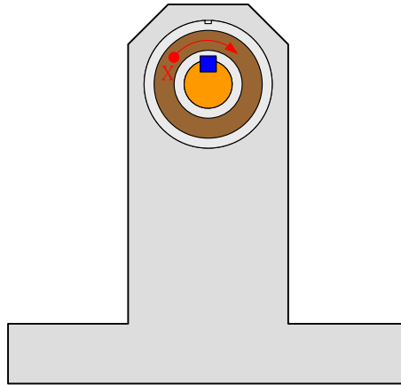
圖 11 單向軸承止逆設計
