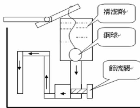
圖[5-3] 為馬桶清潔機構設計草圖
