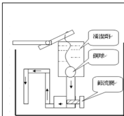
圖[6-1]第一代清潔機構草圖
