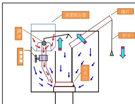
圖[6-3]第二代清潔機構草圖
