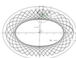
圖二十七(半徑改變)
