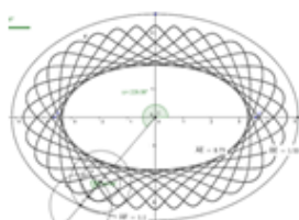
圖二十六(固定半徑)
