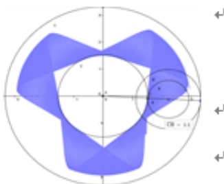
圖十二:模擬圖形↵
