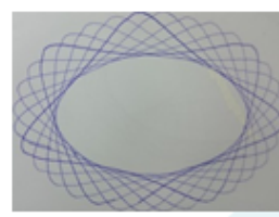
圖二十八(真實圖形)
